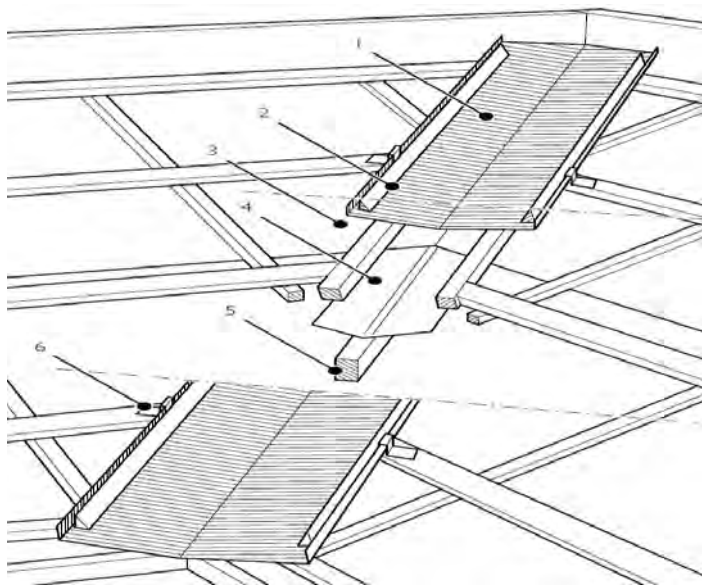
Neelu paigaldamine: 1. Neeluplekk, 2. Neelutihend 3. Aluskate, 4. Neelu alusprofiil, 5. Neelu roovitus 6. Klambrit. Joonis nr 50
